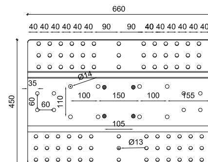
Abbildung 3.4 - Giebelvorrichtung für die Lastverteilung (Cod. 000213) der Vorrichtung LVB/LVBD
