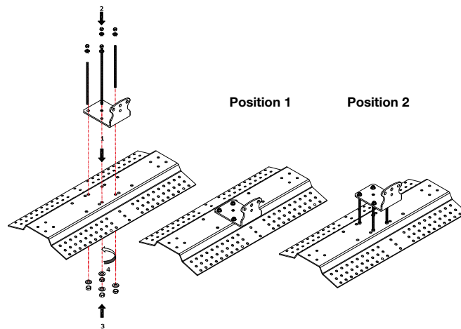
Abbildung 3.5 - Vorrichtung LVB/LVBD mit Lastverteilungsplatte (Cod. 000218)
