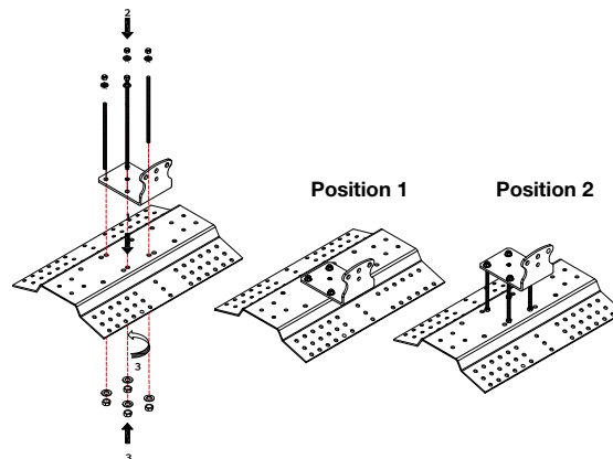
Abbildung 3.6 - Vorrichtung LVB/LVBD mit Lastverteilungsplatte (Cod. 000213)
