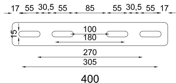
Abbildung 3.8 - Gegenplatte aus verzinktem Stahl (Cod. 000203) der Vorrichtung LVB/LVBD
