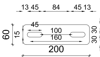
Abbildung 3.7 - Gegenplatte aus verzinktem Stahl (Cod. 000196) der Vorrichtung LVB/LVBD
