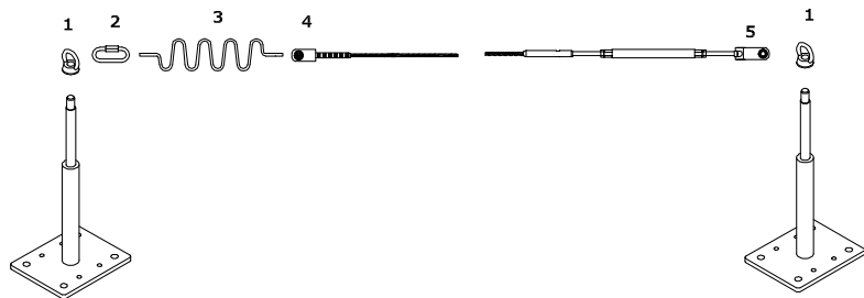
Figure 5.2 - Ligne de vie à une travée
