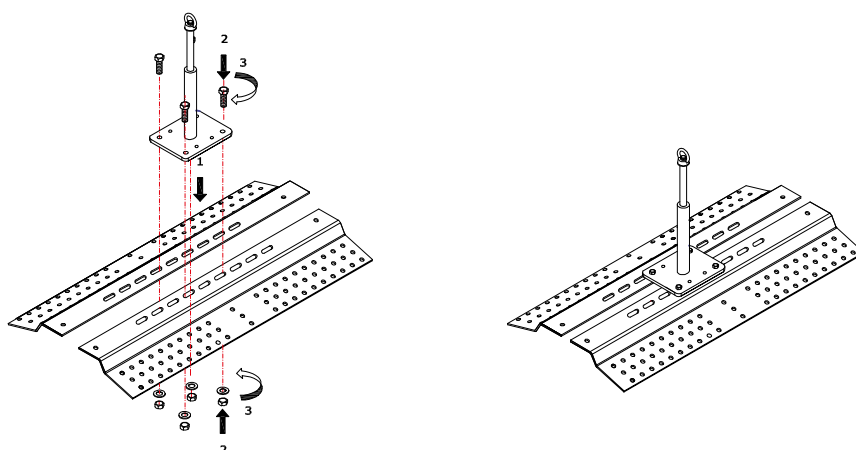
Figure 3.9 - Dispositif PBS avec plaque de répartition pour pente (Code 000220)
