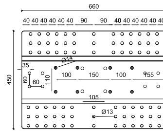
Figure 3.4 - Plaque pour ligne de faîte pour la répartition des charges (Code 000213) du dispositif PBS
