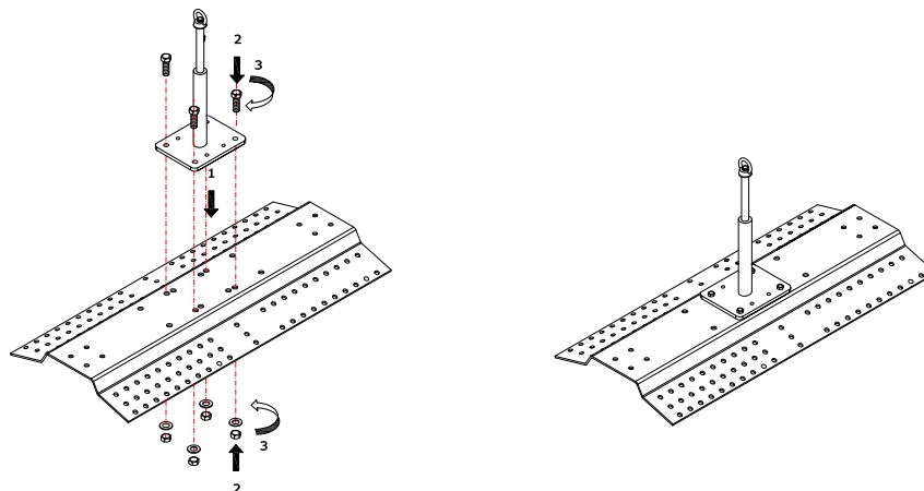
Figure 3.7 - Dispositif PBS avec plaque de répartition pour ligne de faîte (Code 000218)
