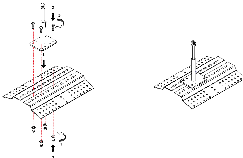
Figure 3.10 - Dispositif PBS avec plaque de répartition pour pente (Code 000224)
