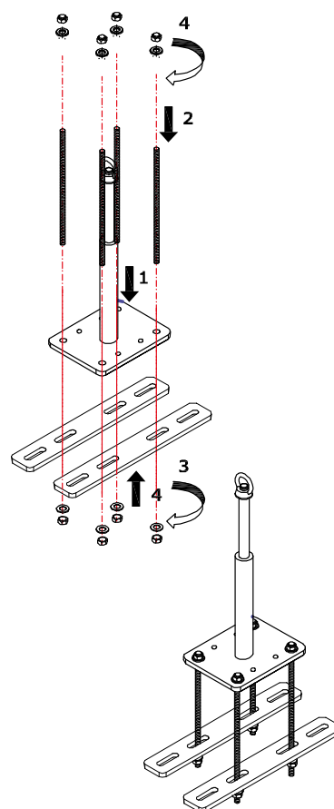
Figura 3.16 - Dispositif PBS/PBSC avec contre-plaques (Code 000203)
