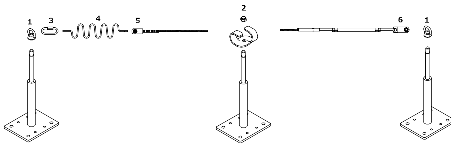
Figure 5.3 - Ligne de vie à deux travées
