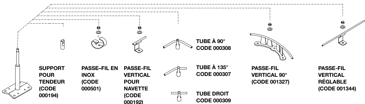
Figure 4.30 - Potelet PBS/PBSC pouvant être associé à un des accessoires suivants :
