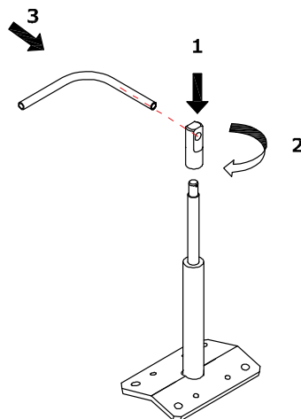
Figure 4.32 - PBS/PBSC – Assemblage avec passe-fil et tube
