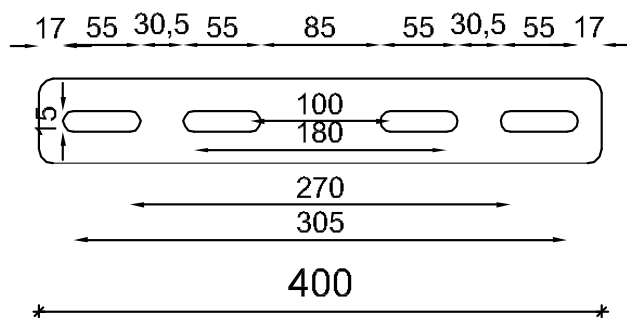
Figure 3.13 - Contre-plaque en acier galvanisé (Code 000203) pour les dispositifs PBS/PBSC
