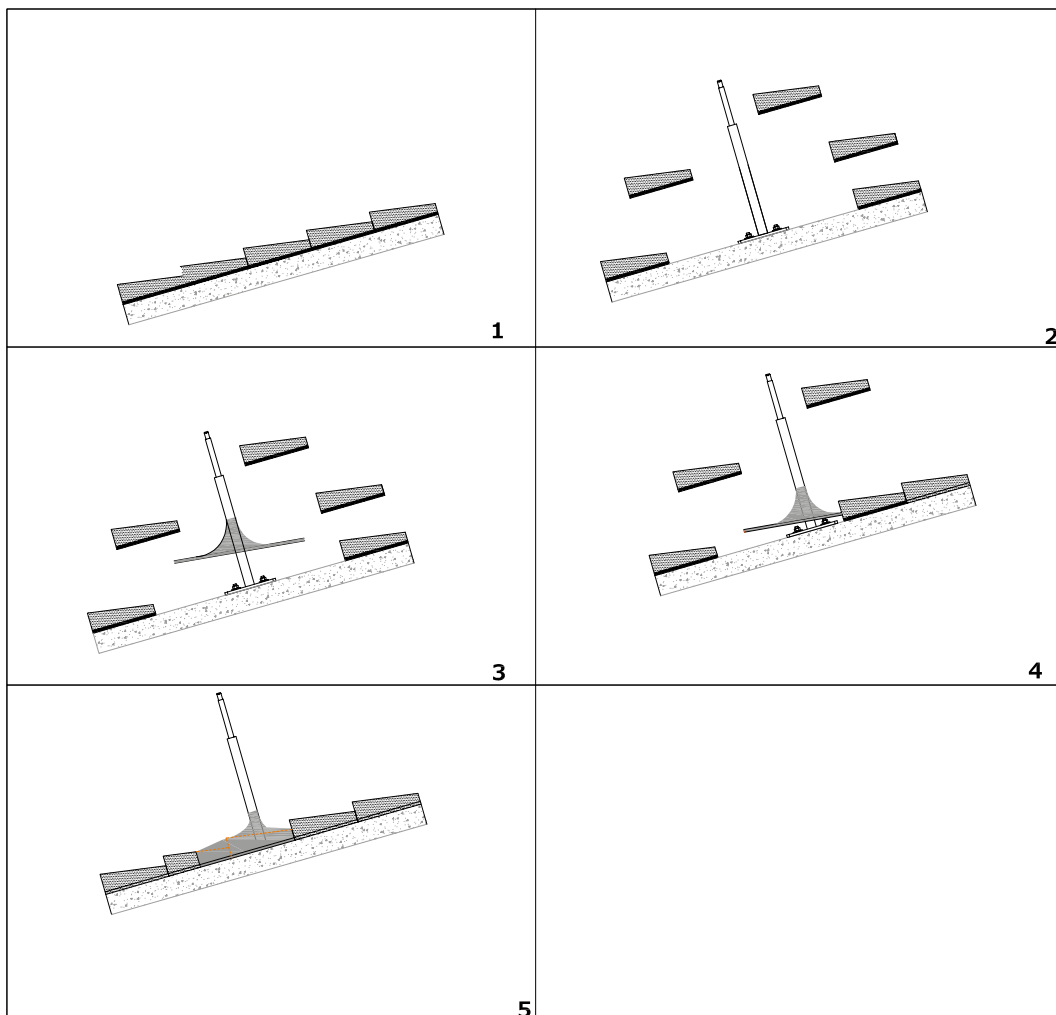
Figure 3.17 – Imperméabilisation du potelet PBS/PBSC
