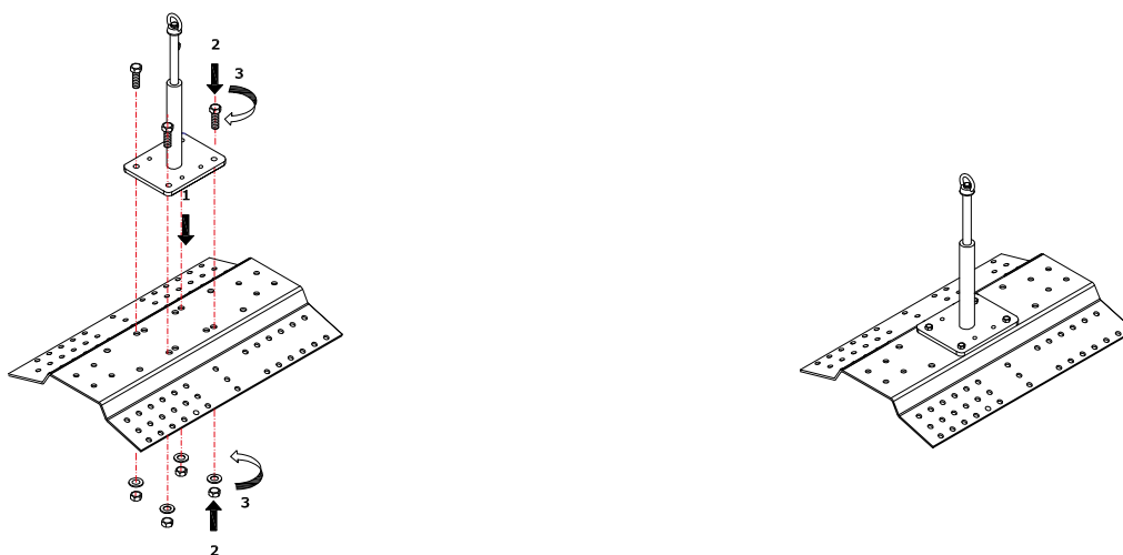
Figure 3.8 - Dispositif PBS avec plaque de répartition pour ligne de faîte (Code 000213)
