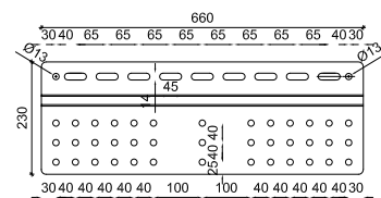
Figure 3.6 - Plaque pour pente pour la répartition des charges (Code 000224) du dispositif PBS
