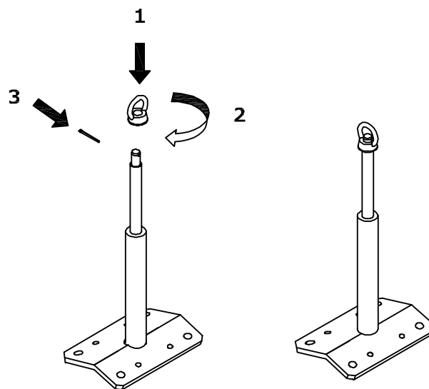
Figure 4.29 - Assemblage du potelet PBS/PBSC avec œillet et goupille (Code 000058)
