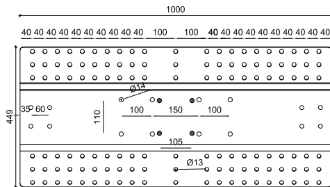
Figure 3.3 - Plaque pour ligne de faîte pour la répartition des charges (Code 000218 ) du dispositif PBS
