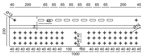
Figure 3.5 - Plaque pour pente pour la répartition des charges (Code 000220) du dispositif PBS
