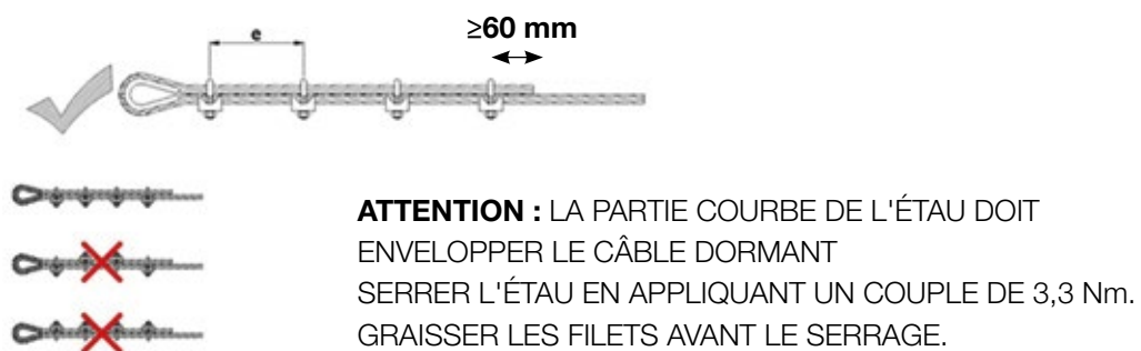
Figure 5.4 - Positionnement du câble avec les étaux
