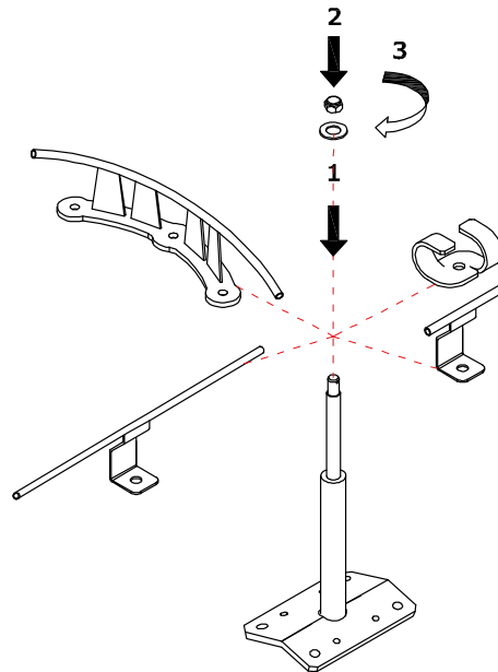
Figure 4.31 - Potelet PBS/PBSC avec accessoires et écrou de sécurité
