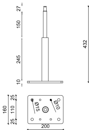
Figura 3.1 - Palo PBS
