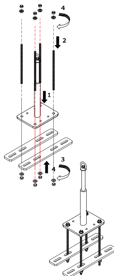
Figura 3.16 - Dispositivo PBS/PBSC con contropiatti (Cod. 000203)
