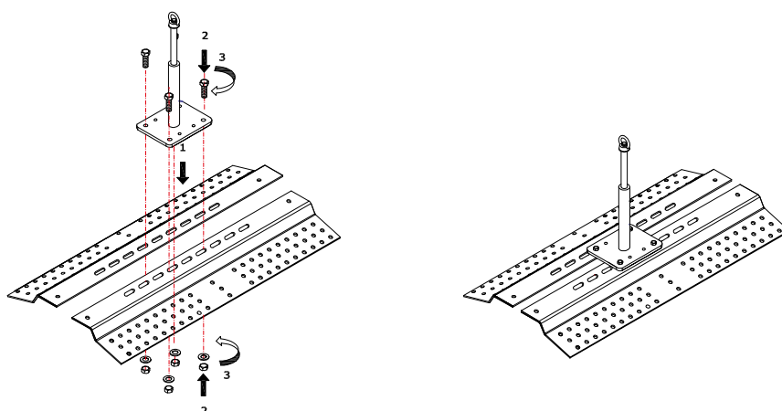
Figura 3.9 - Dispositivo PBS con piastra di ripartizione da falda (Cod. 000220)
