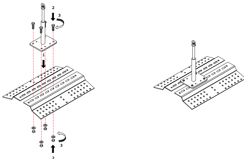
Figura 3.10 - Dispositivo PBS con piastra di ripartizione da falda (Cod. 000224)
