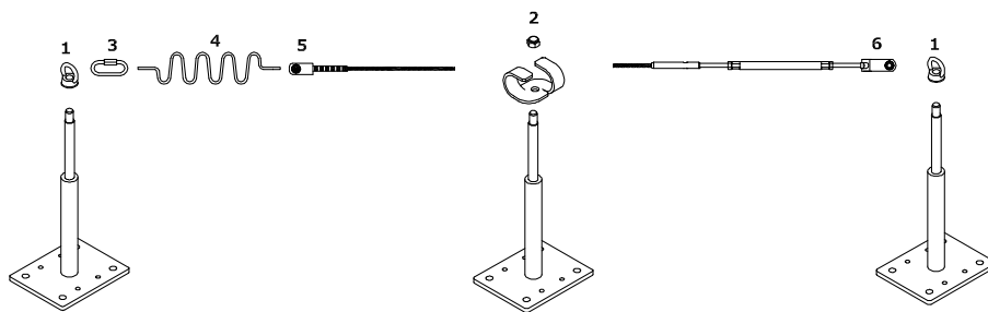
Figura 5.3 - Linea vita a due campate
