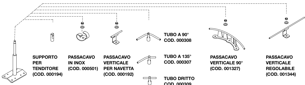
Figura 4.30 - Palo PBS/PBSC combinabile con uno dei seguenti accessori:
