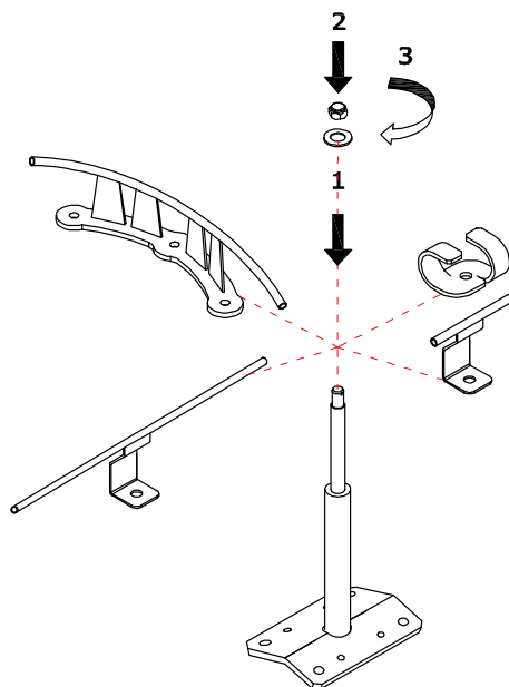
Figura 4.31 - Palo PBS/PBSC con accessori e dado autobloccante
