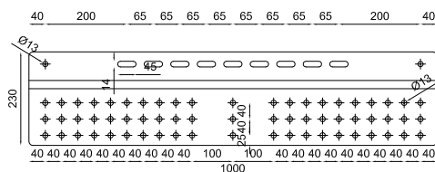
Figura 3.5 - Piastra da falda per ripartizione carichi (Cod. 000220) del dispositivo PBS
