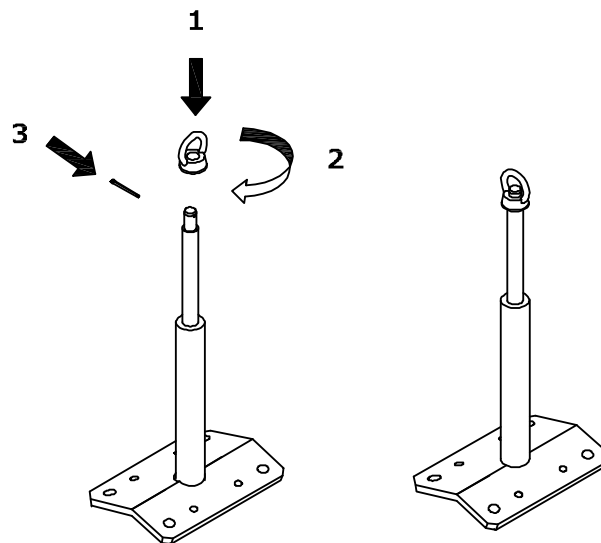
Figura 4.29 - Assemblaggio del palo PBS/PBSC con golfare e copiglia (Cod. 000058)
