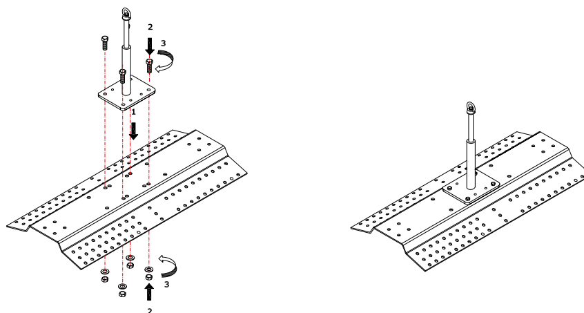
Figura 3.7 - Dispositivo PBS con piastra di ripartizione da colmo (Cod. 000218)
