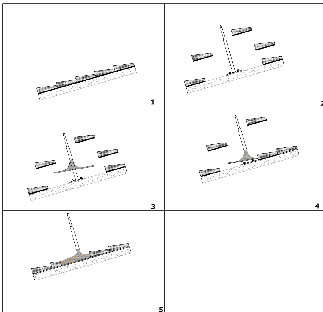
Figura 3.17 – Impermeabilizzazione del palo PBS/PBSC
