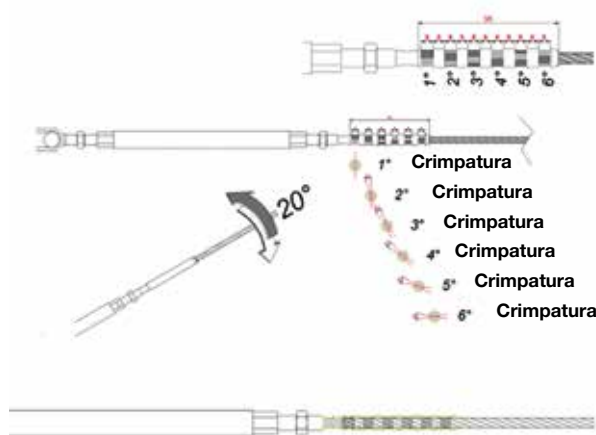
Figura 5.1 - Crimpatura
