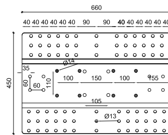
Figura 3.4 - Piastra da colmo per ripartizione carichi (Cod. 000213) del dispositivo PBS
