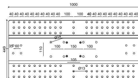
Figura 3.3 - Piastra da colmo per ripartizione carichi (Cod. 000218 ) del dispositivo PBS
