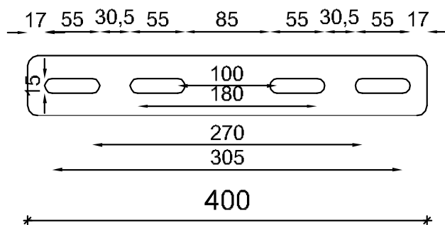
Figura 3.13 - Contropiatto in acciaio zincato (Cod. 000203) per dispositivi PBS/PBSC
