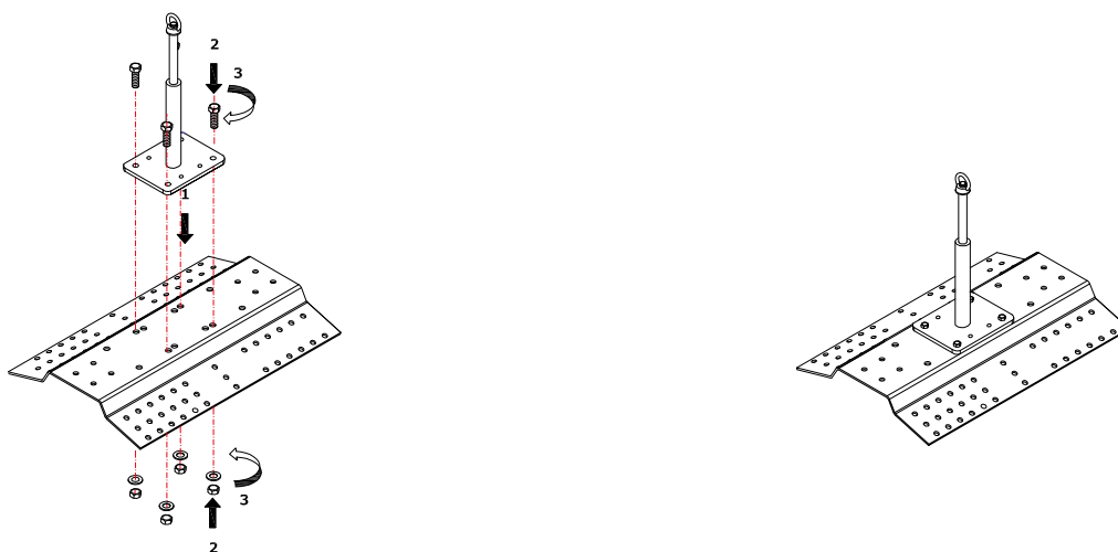
Figura 3.8 - Dispositivo PBS con piastra di ripartizione da colmo (Cod. 000213)
