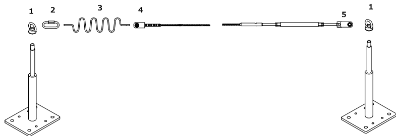
Figura 5.2 - Linea vita a una campata
