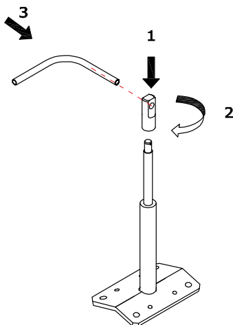
Figura 4.32 - PBS/PBSC – Assemblaggio con passacavo e tubo
