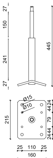
Figura 3.2 – Palo PBSC
