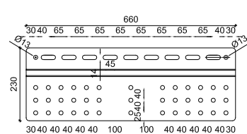
Figura 3.6 - Piastra da falda per ripartizione carichi (Cod. 000224) del dispositivo PBS
