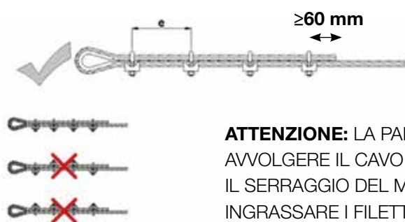
Figura 5.4 - Posizionamento cavo con morsetti
