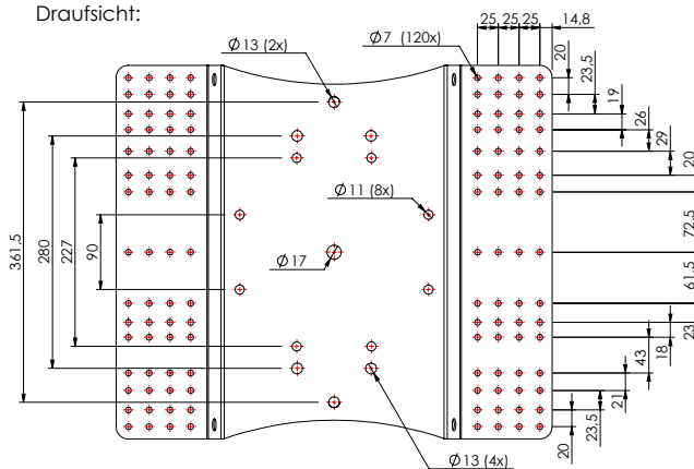
Draufsicht:
